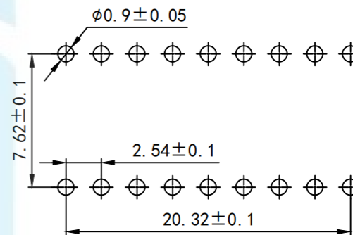
PCB开孔
