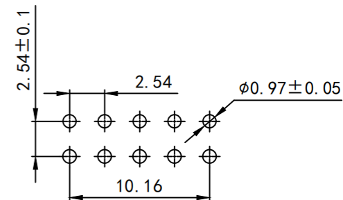
PCB开孔
